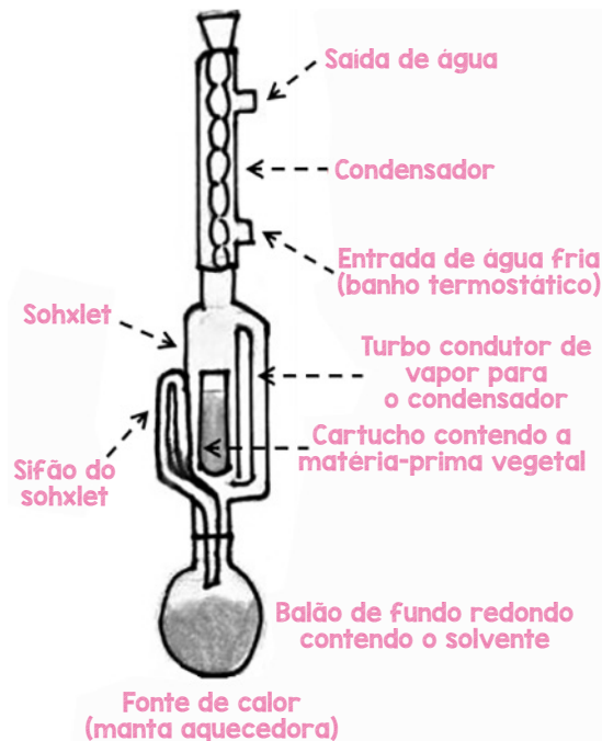
Figura 3. Extrator do tipo sohxlet
